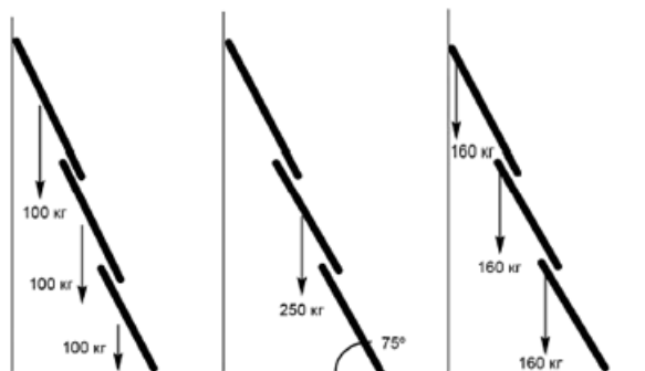
Рисунок 8 - Схемы испытаний выдвжной лестницы в рабочем положении на прочность
