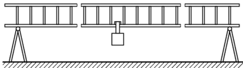
Рисунок 2 - Схема подвески контрольного груза
