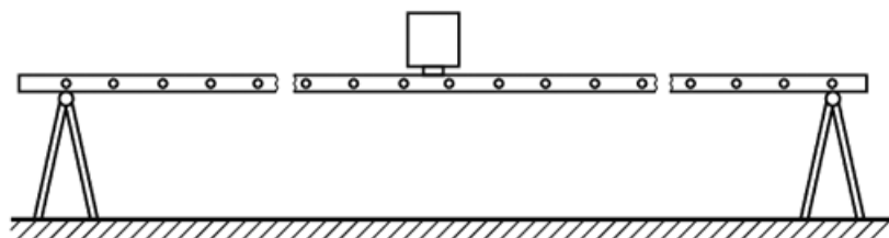
Рисунок 1 - Схема установки лестницы на опоры
