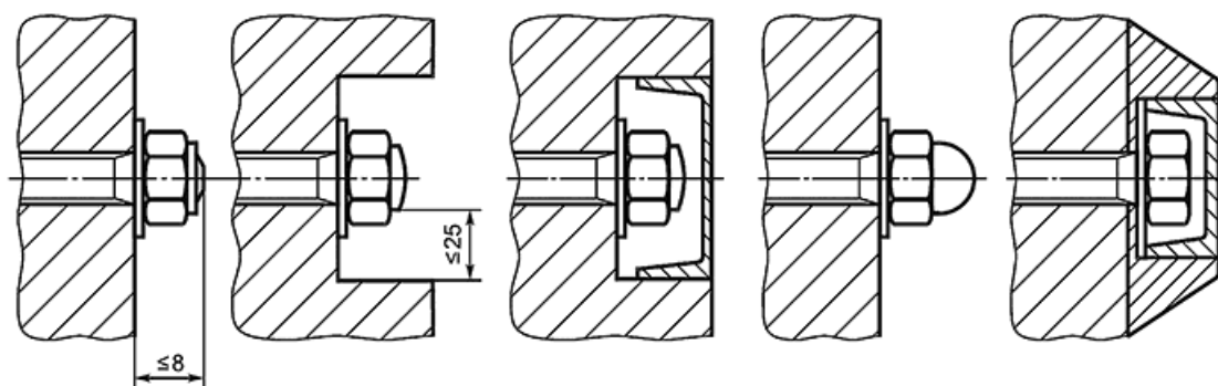
а) Примеры защиты соединений
