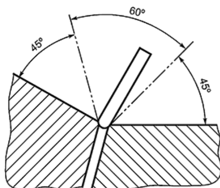
Рисунок А.5 - Пример проведения испытания по А.4.2
