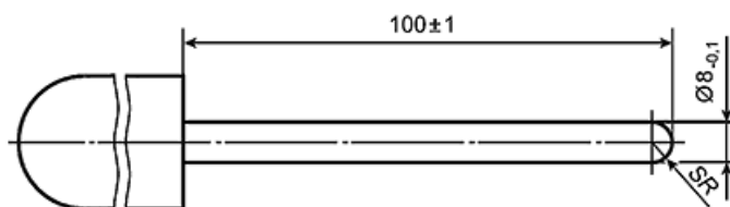
а) Круглый стержень диаметром 8 мм
