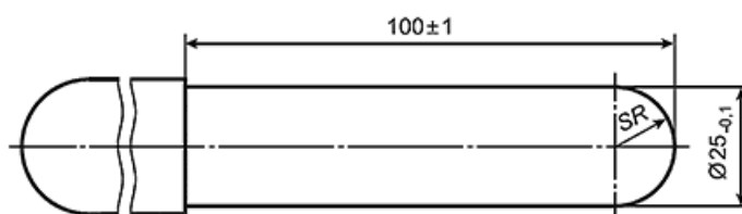
б) Круглый стержень диаметром 25 мм
