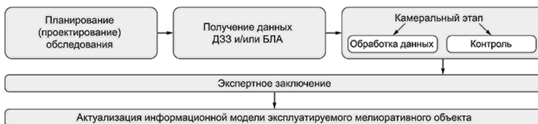
Рисунок 2 - Этапы мониторинга технического и экологического состояния ГМС или ГТС методами ДЗЗ из космоса и/или БЛА
